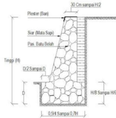
Gambar 5. Sistem penahan dinding batu kali yang diterapkan
