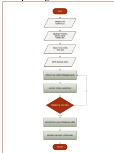
Gambar 3. Flowchart Aplikasi
