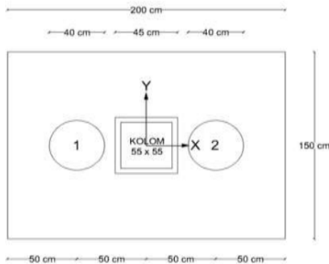
Gambar 8 Tampak Atas Kelompok 2 tiang
