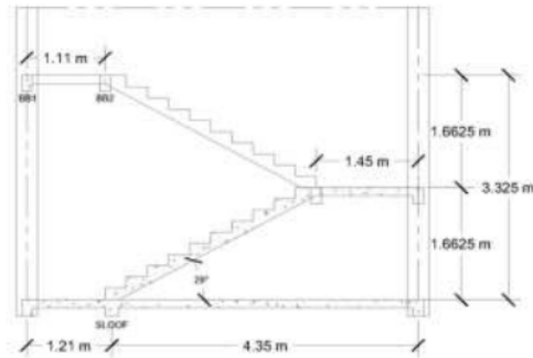
Gambar 6 potongan tangga tampak samping
