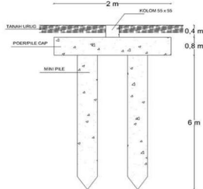
Gambar 9 Potongan Kelompok Tiang Arah X Maka menggunakan base plate dengan ukuran 500x500x20 mm
