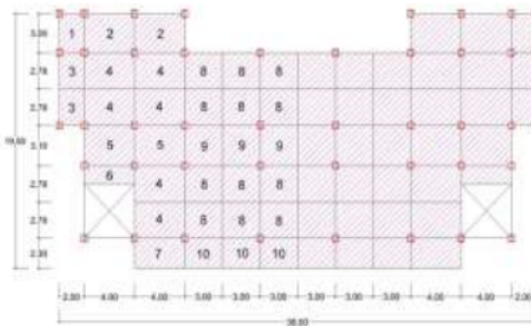
Gambar 4 Denah Pelat Lantai 2
