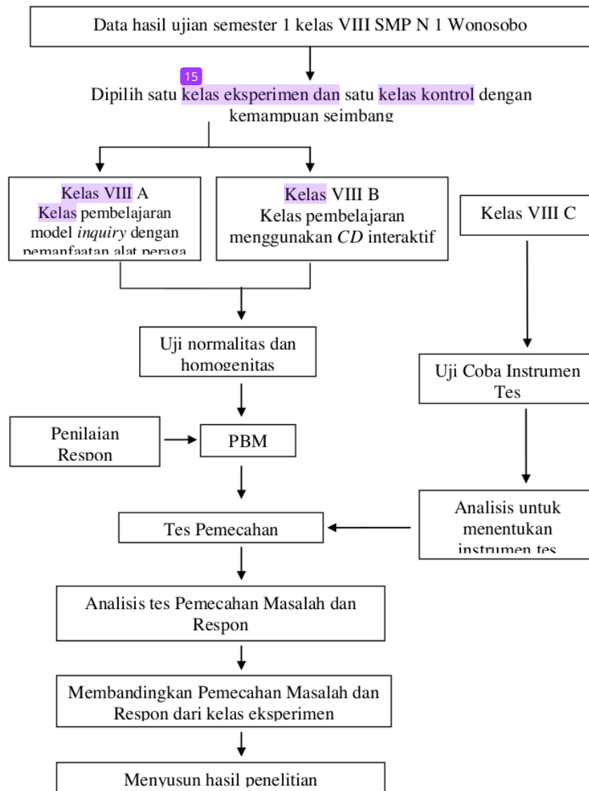
Gambar 1. Desain Penelitian
