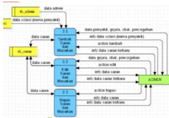
Gambar 9. DFD Level 1 Proses 3.0 Saran dan Masukan
