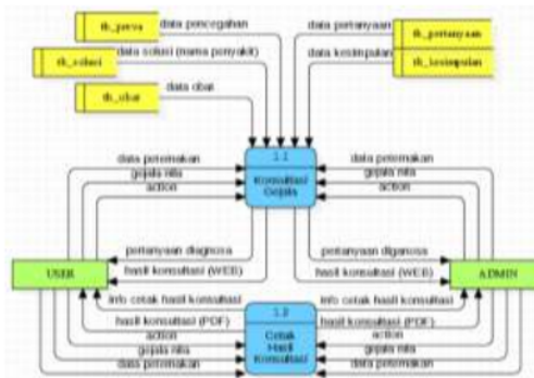
Gambar 7. DFD Level 1 Proses 1.0 Konsultasi
