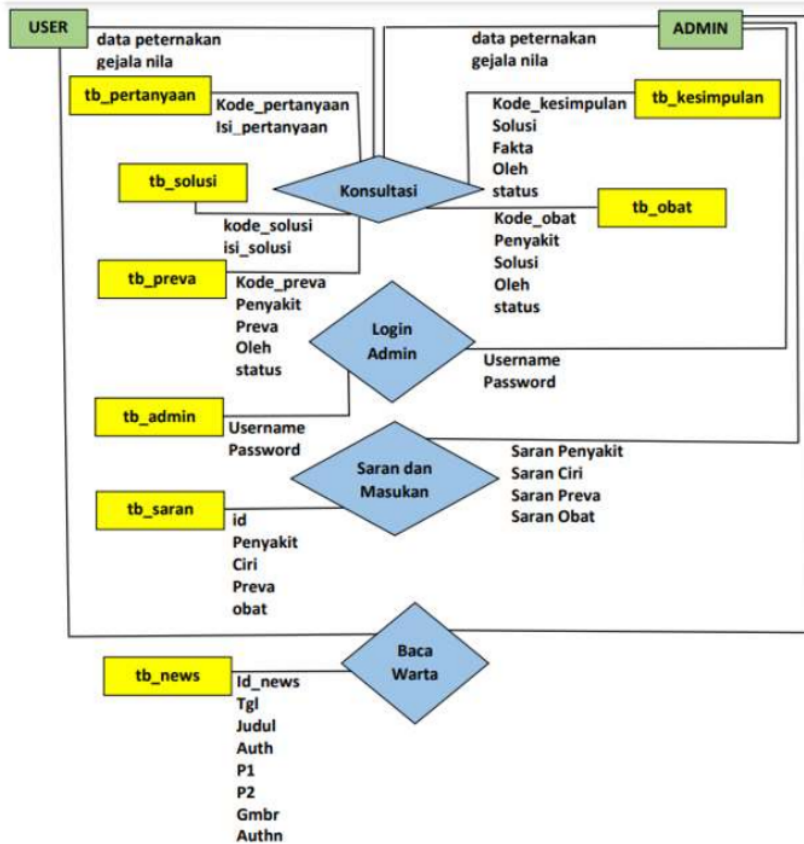
Gambar 11. ER Diagram
