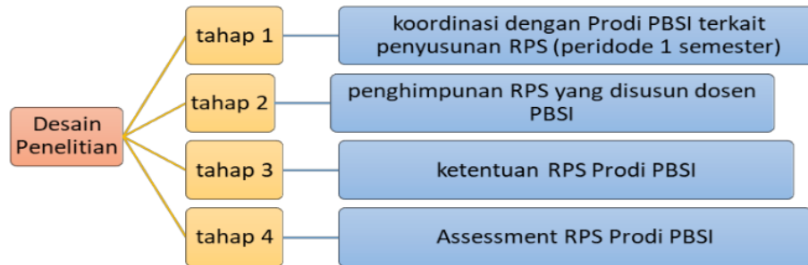
Gambar 2. Desain Penelitian
