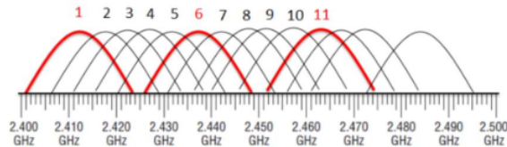
Gambar 3. Grafik kanal WiFi [3]
