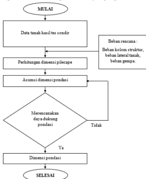
Gambar 6 Bagan Alir Perhitungan Pondasi. Pada gambar 2 dijelaskan tahapan perhitungan pondasi Perencanaan Struktur Museum Permainan Anak Tradisional Di Bringin Kecamatan Ngaliyan.
