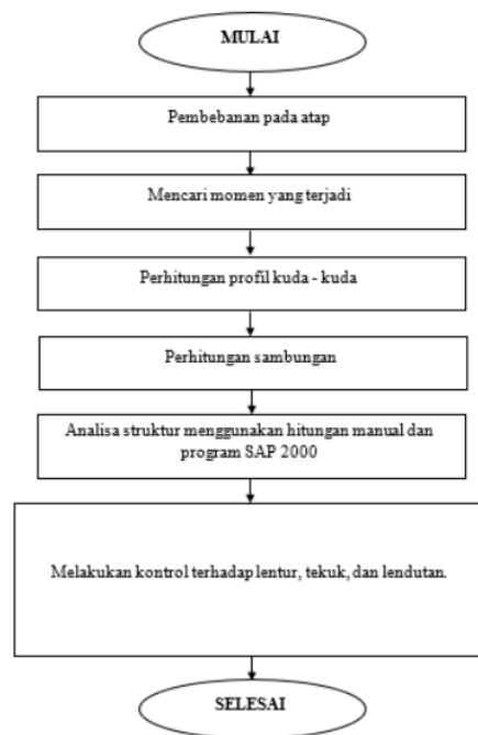
Gambar 2 Bagan Alir Perhitungan atap.
