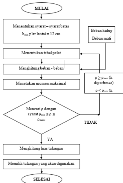
Gambar 3 Bagan Alir Perhitungan Pelat.
