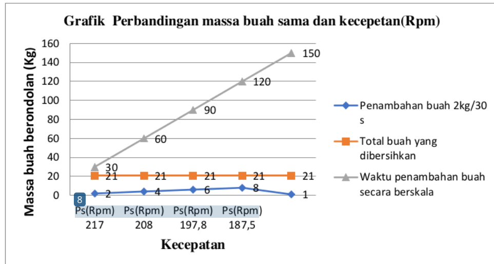
Gambar 14. Perbandingan massa buah dan kecepatan
