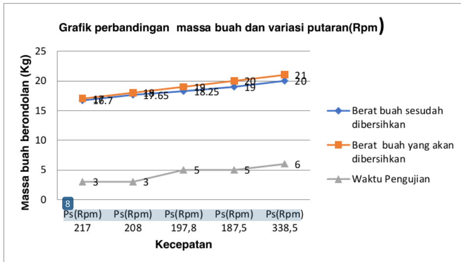
Gambar 13. Perbandingan massa buah dan variasi putaran Menggunakan variasi putaran sangat mempengaruhi hasil akhir kualitas
