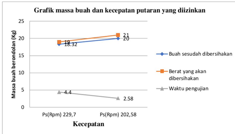
Gambar 15. Massa buah dan kecepatan putaran yang diizinkan
